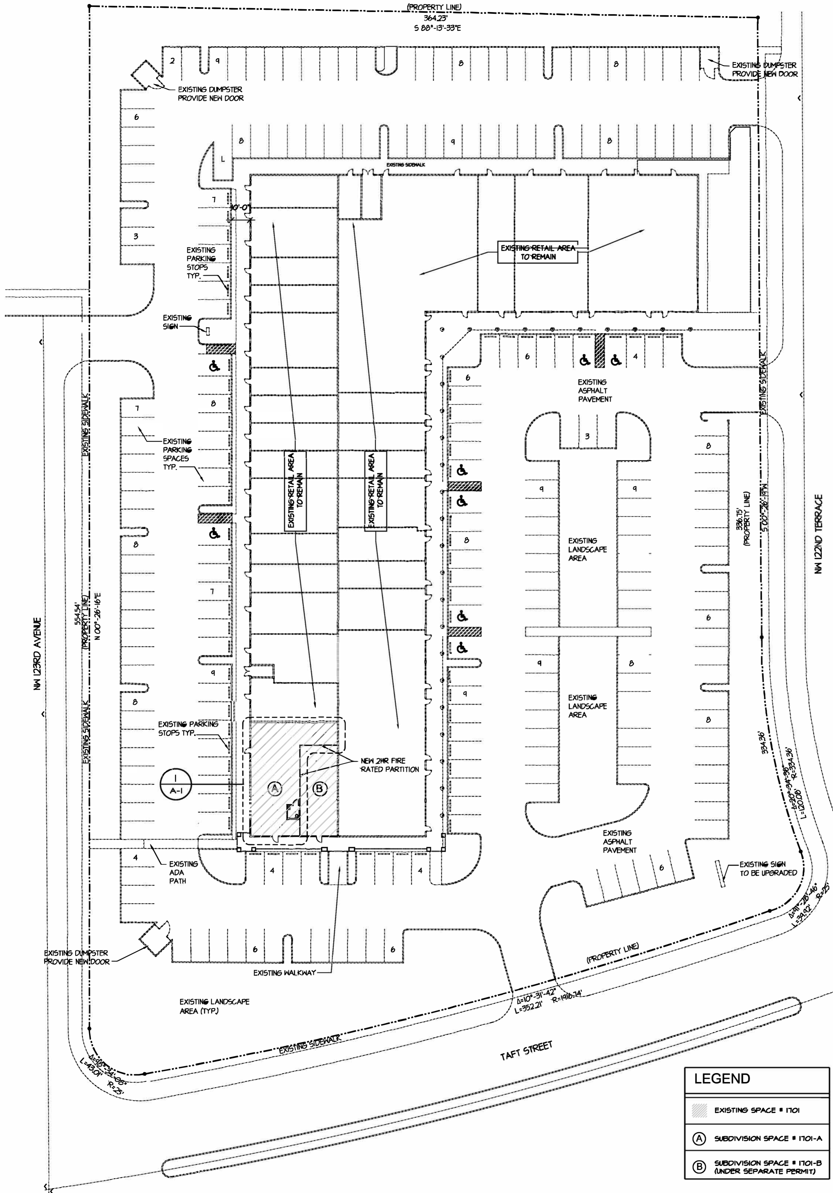
SITE/FLOOR PLAN SCALE: 1" = 30'-0"
